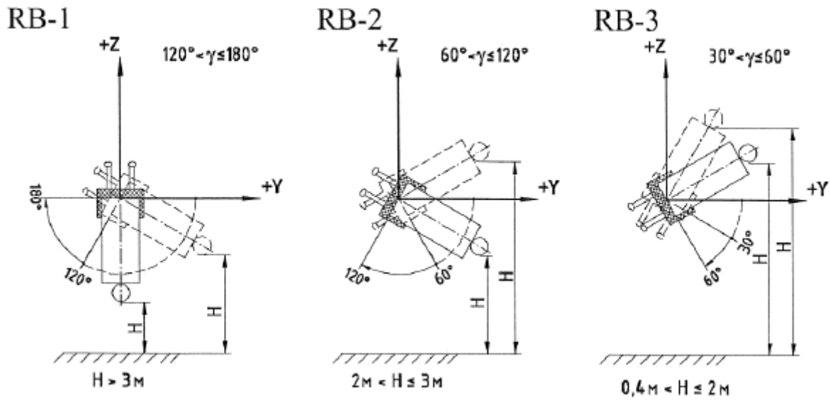
Рис. 3. Наклон пассажирских кресел набок
