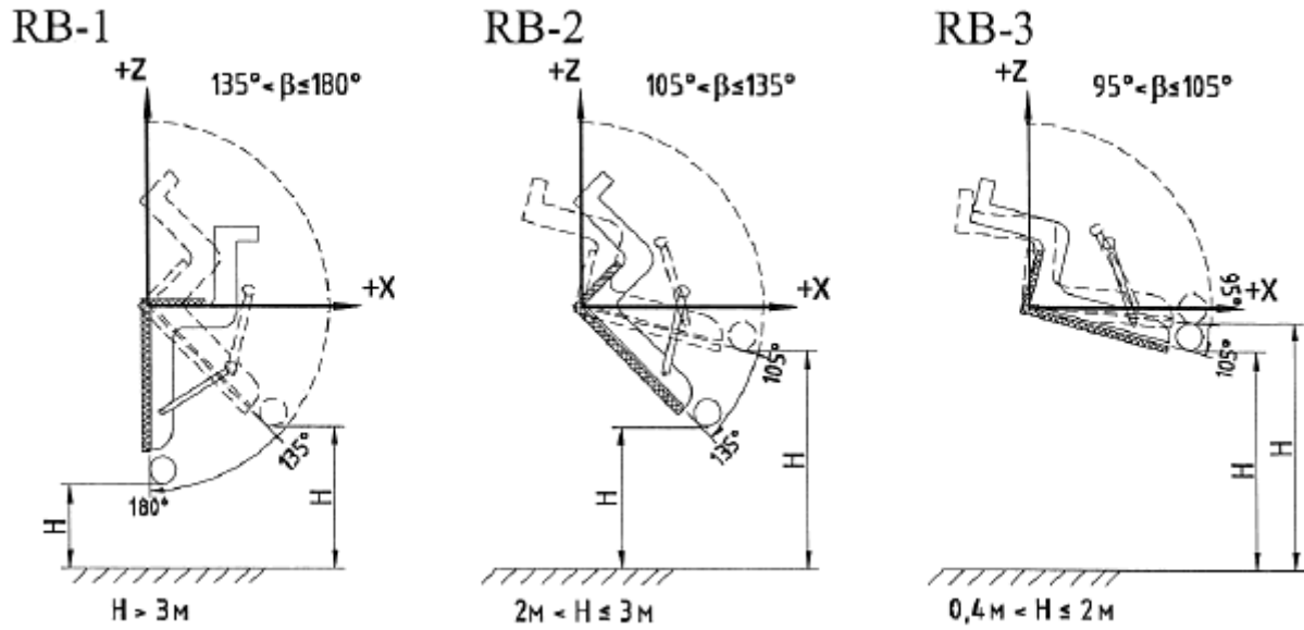
Рис. 2. Наклон пассажирских кресел назад Виды наклона пассажирских кресел набок представлены на рисунке 3.
