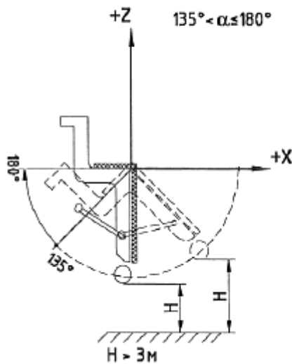
Рис. 1. Наклон пассажирских кресел вперед Виды наклона пассажирских кресел назад представлены на рисунке 2.
