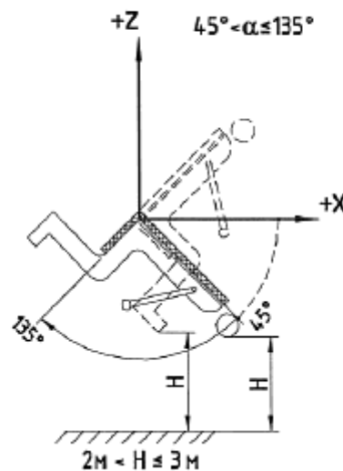
Рис. 1. Наклон пассажирских кресел вперед Виды наклона пассажирских кресел назад представлены на рисунке 2.
